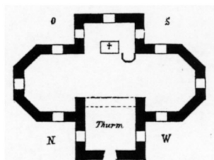
Kirchengrundriß n. Schmidt 1889
